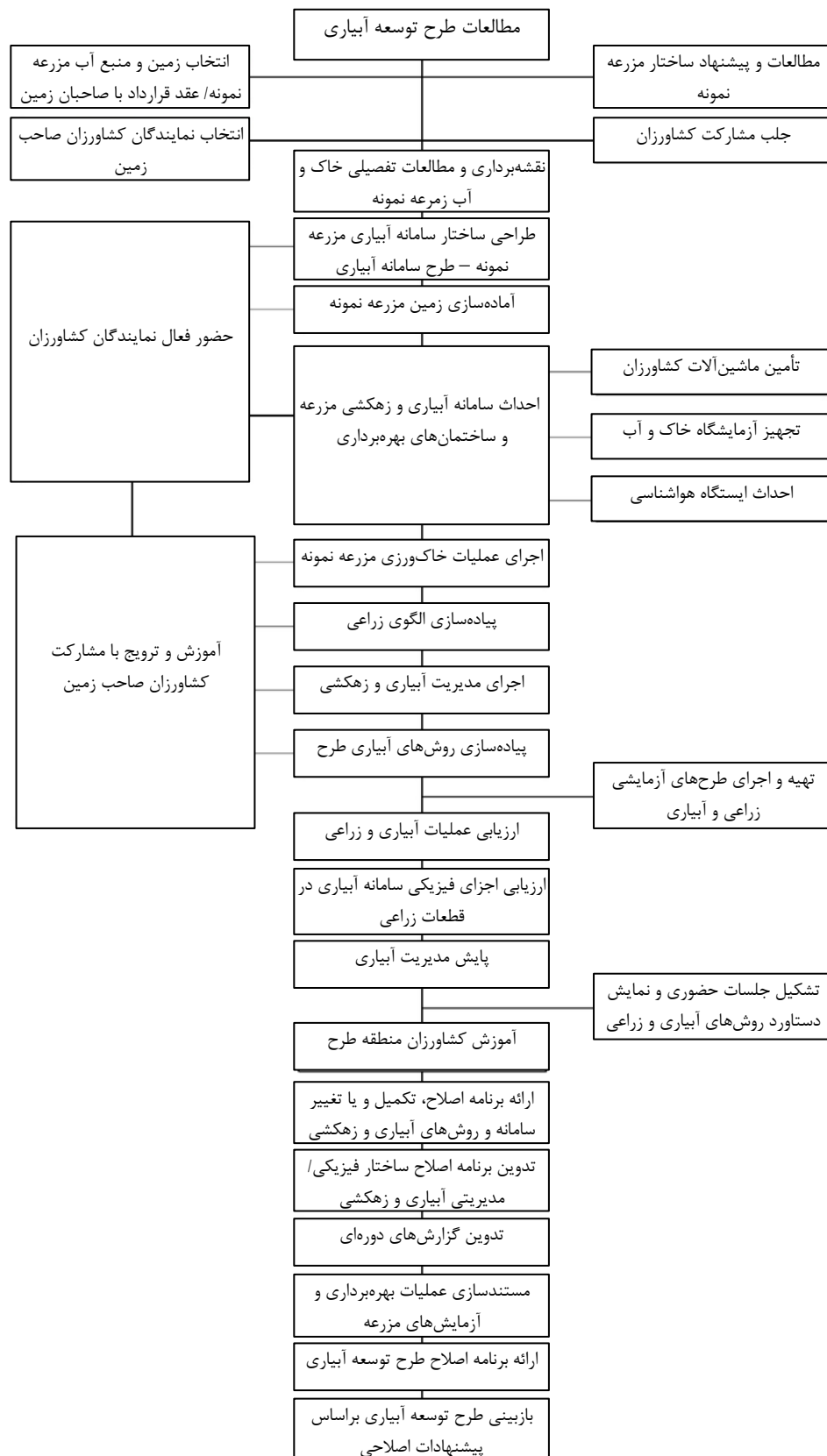
شکل ۳-۱- خلاصه روند انجام مراحل برنامه‌ریزی، طراحی، ساخت و بهره‌برداری مزرعه نمونه
