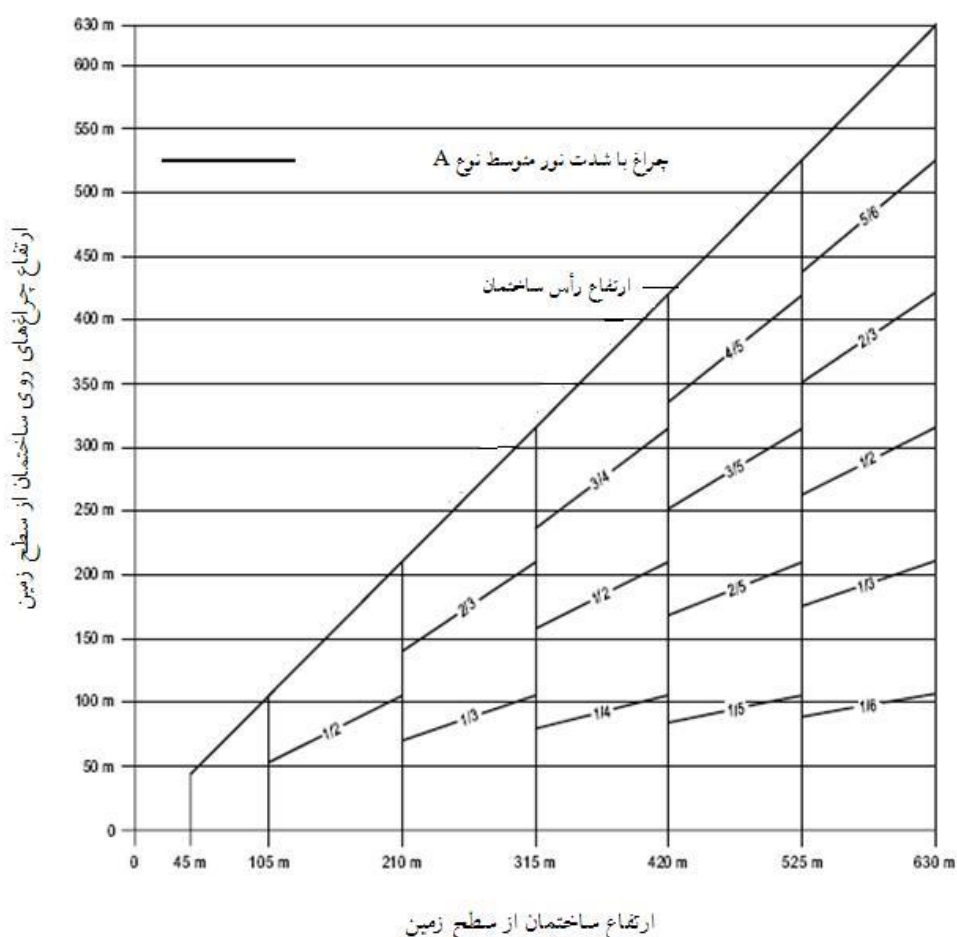
شکل ۳-۱۰- مکان قرارگیری سامانه چراغ‌های چشمک‌زن سفید با شدت نور متوسط نوع A
