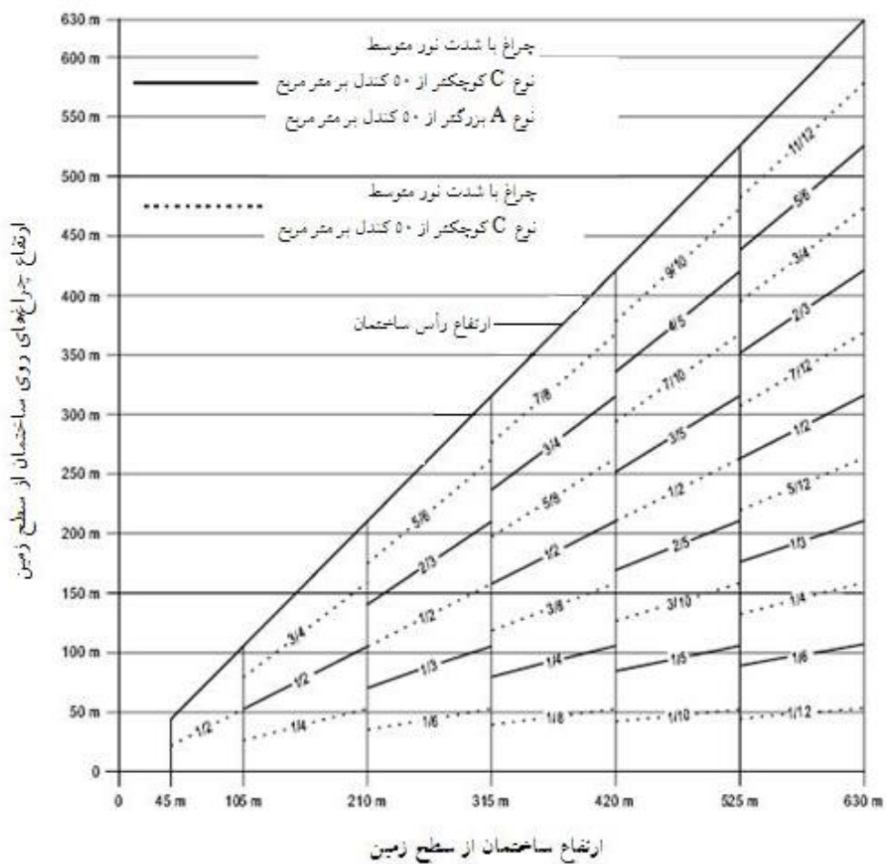
شکل ۳-۱۴- مکان قرارگیری سامانه چراغ‌های دوتایی با شدت نور متوسط نوع A \ نوع C
