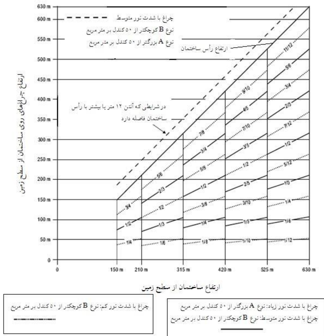
شکل ۳-۱۶- مکان قرارگیری سامانه چراغ‌های دوتایی با شدت نور متوسط، زیاد، نوع A \ نوع B
